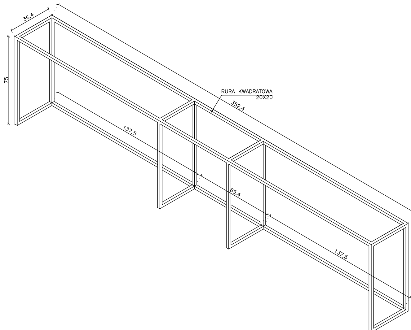
STALOWA KONSTRUKCJA NÓŻEK - IZOMETRIA
