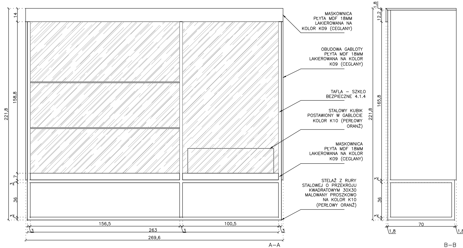
WIDOK Z PRZODU
