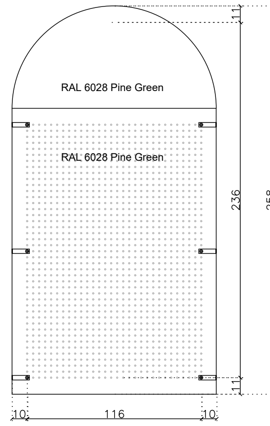
OKIENNICA WIDOK SALA 02
