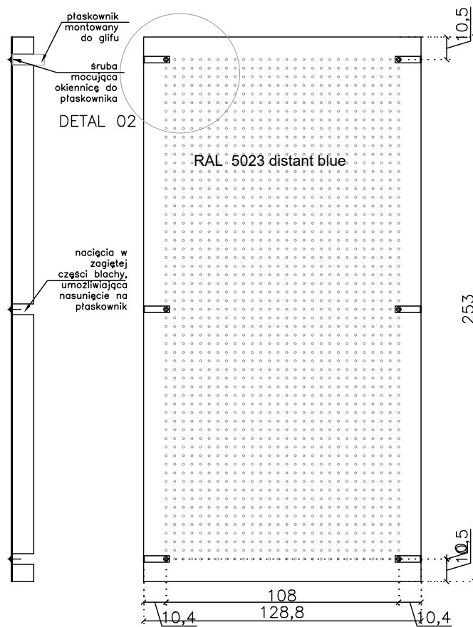
OKIENNICA WIDOK SALA 01
