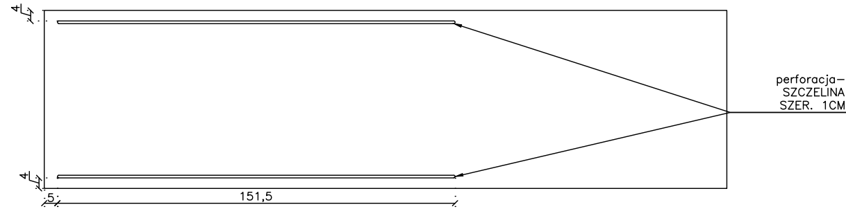
WIDOK Z GÓRY NA DNO GABLOTY
